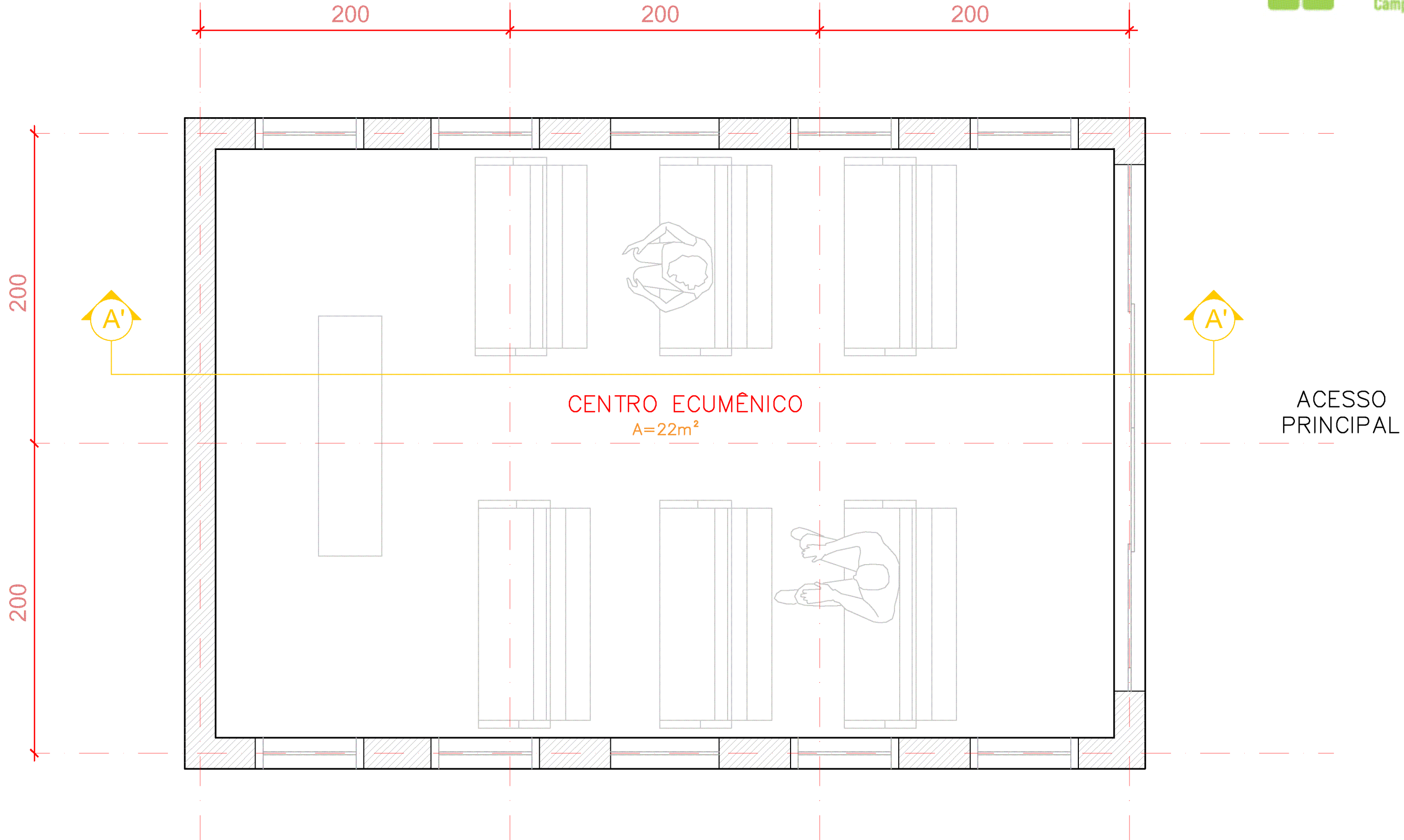
Planta Baixa - Centro Ecumênico Esc.: indicada
