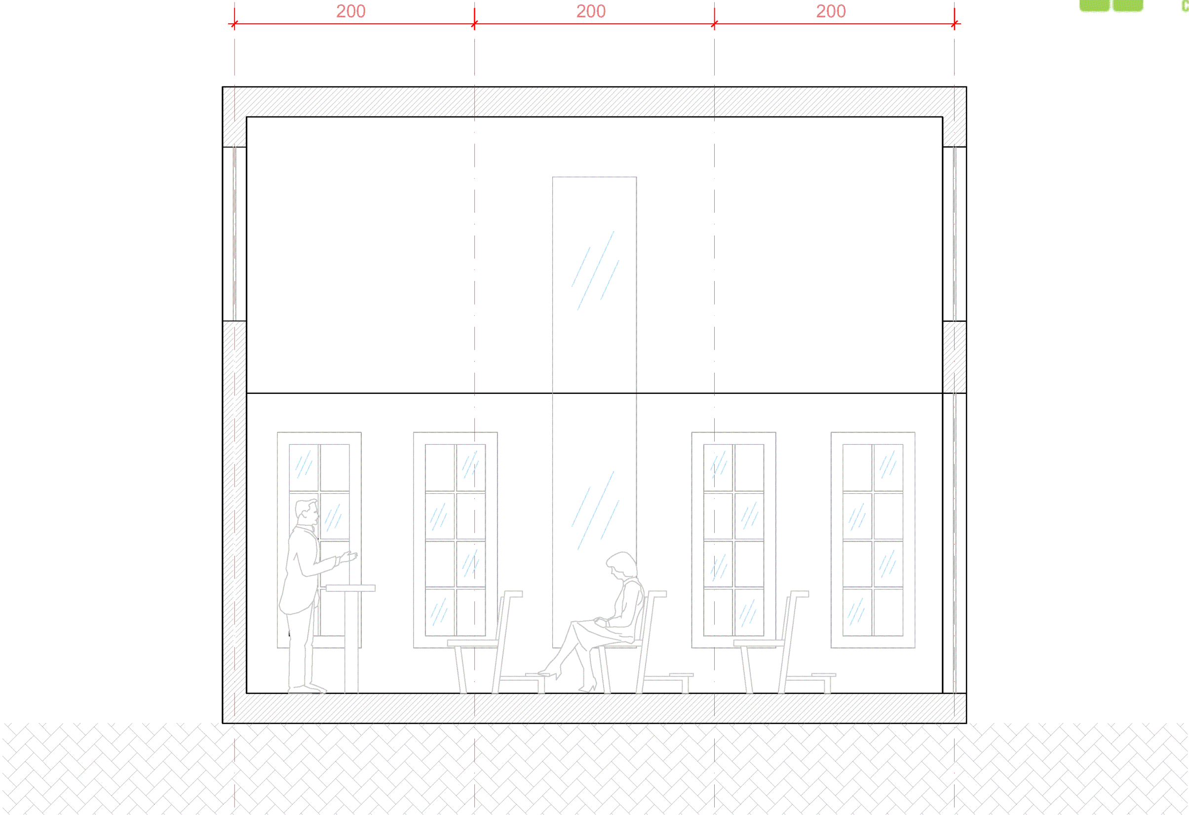
Corte AA' - Centro Ecumênico Esc.: indicada
